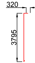
პოზ. 1 Ø16; A500C
